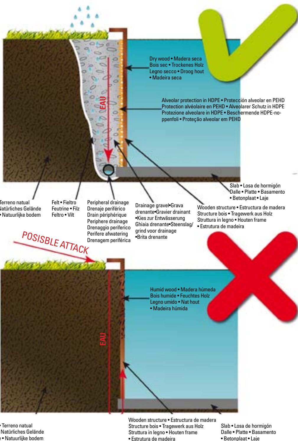
Alveolar protection in HDPE Protección alveolar en PEAD Protection alvéolaire en PEHD Alveolar Schutz in PEHD Protezione alveolare in PEAD Beschermente HDPE-noppenfoli Proteção alveolar em PEAD
